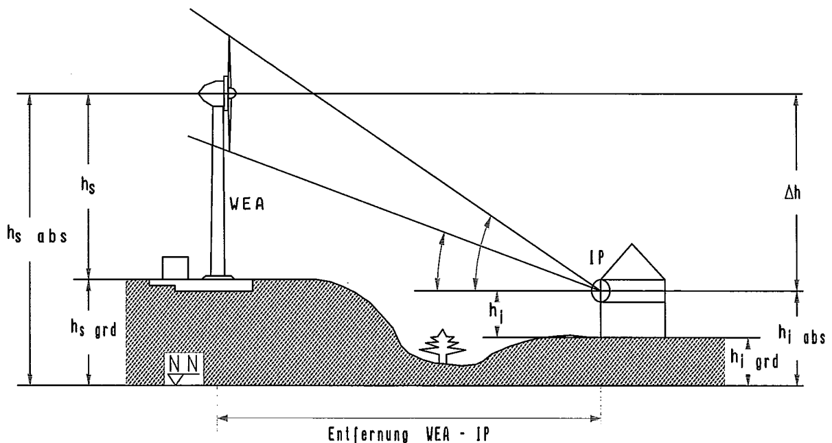
Bild 3: Geometrische Verhältnisse, Vertikalschnitt
