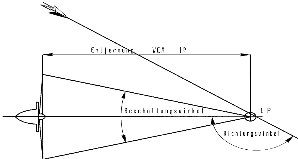
Bild 2: Geometrische Verhältnisse; Draufsicht
